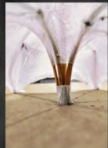
COLOCACIÓN DE MEMBRANA EN ESTRUCTURA CON TEMPLADORES
